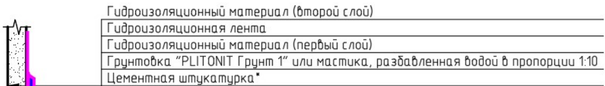
Разрез 1-1
